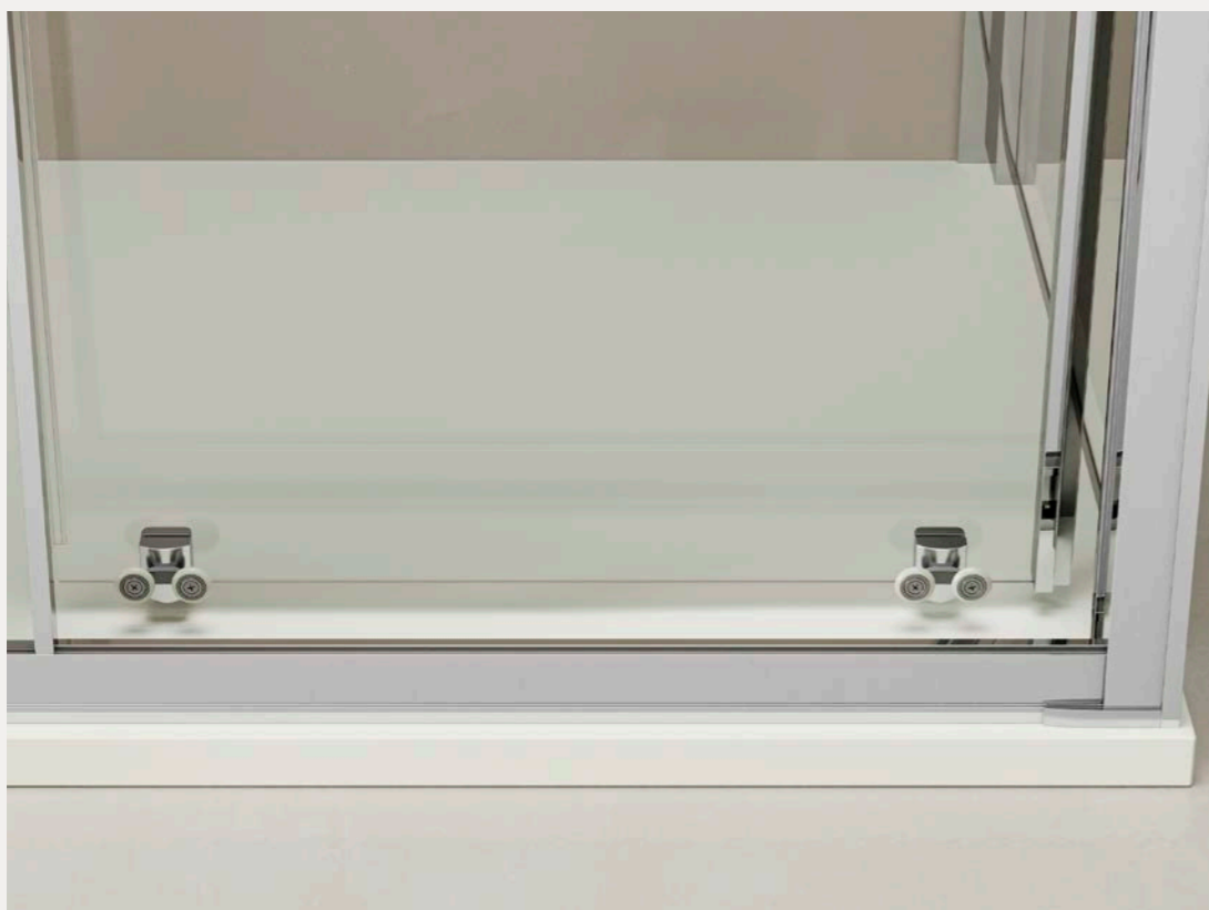
gruppo di scorrimento regolabile con doppio cuscinetto a sfera sistema di sgancio rapido applicato direttamente all'anta
